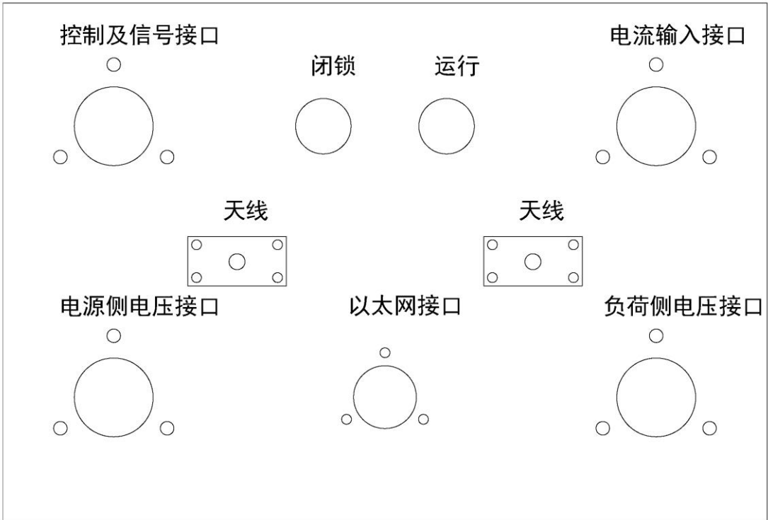
图 2.5-2 装置底部布置图
