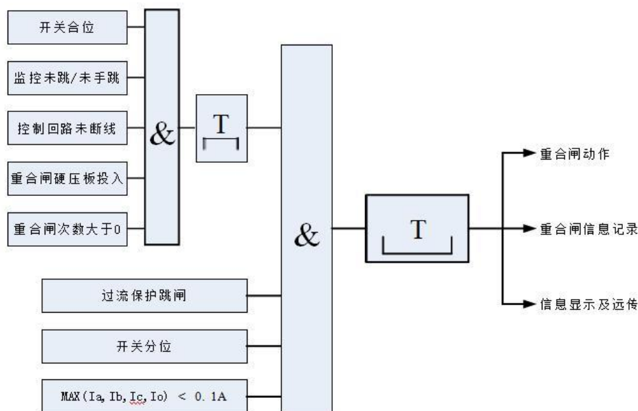
图 4.2-3 相电流重合闸逻辑图
