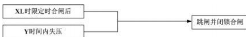
图 4.3-7 闭锁合闸逻辑图
