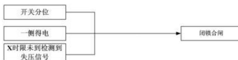
图 4.3-3X 时限闭锁(瞬压闭锁)逻辑图
