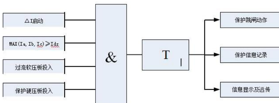
图 4.2-1 过流保护逻辑图
