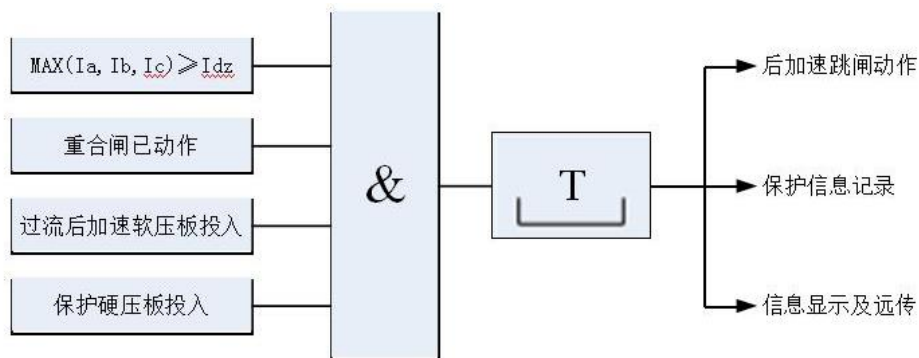
图 4.2-4 过流后加速保护逻辑图
