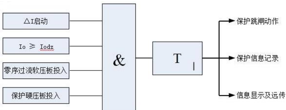
图 4.2-2 零序电流过流保护逻辑图
